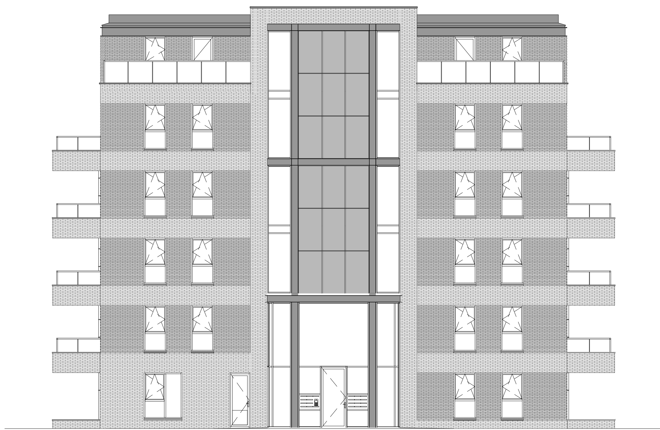
Noordwest - voorgevel
